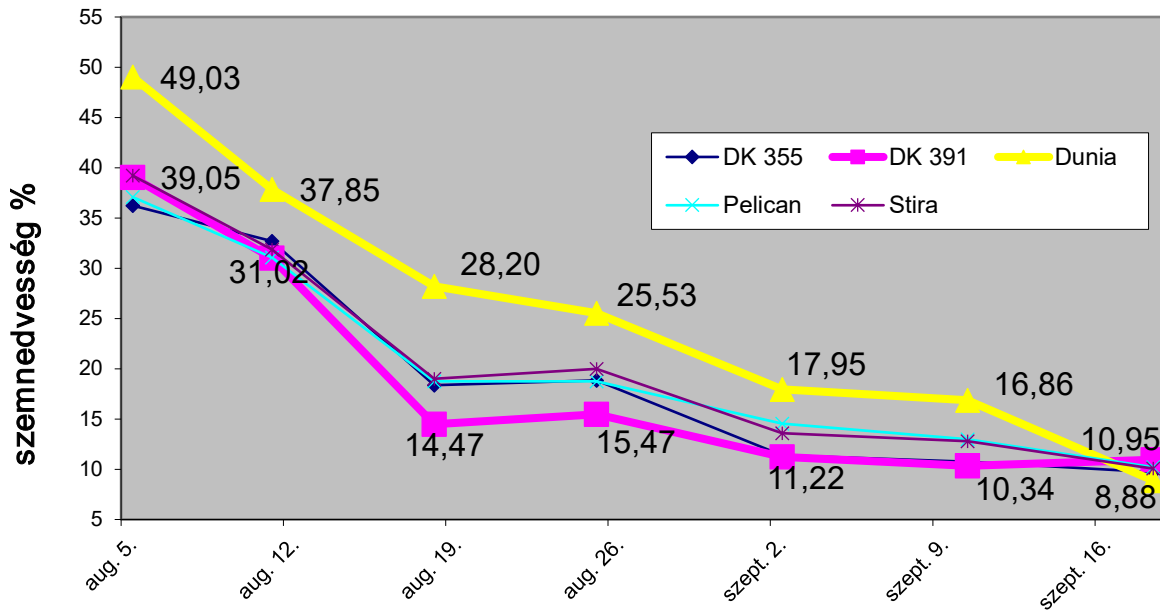
2. ábra: Éréscsoport sztenderd hibridek szemnedvesség leadási görbéje, 2003, korai csoport, Iregszemcse, OMMI).
